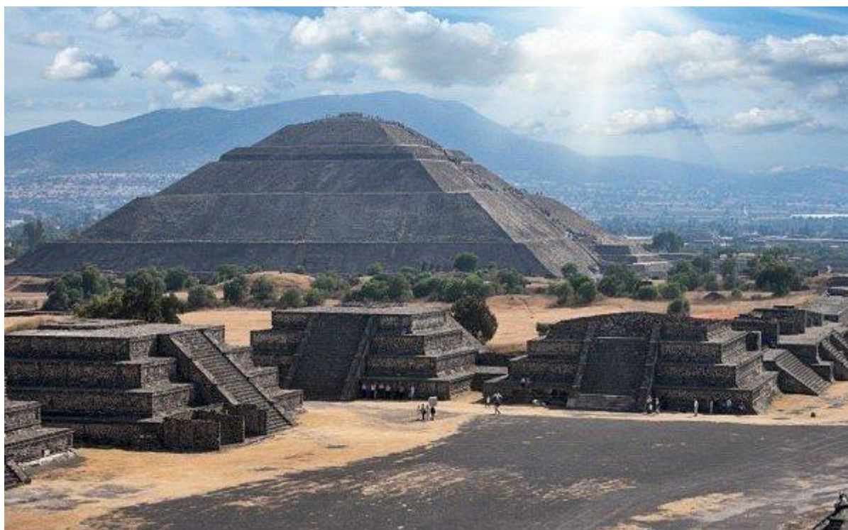
Obr.4:Aztécká pyramida
